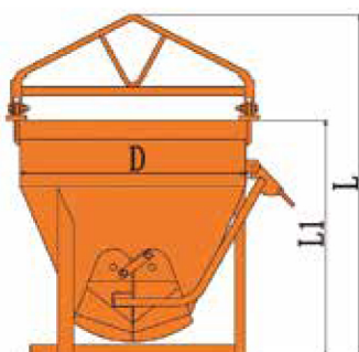
■寸法図
